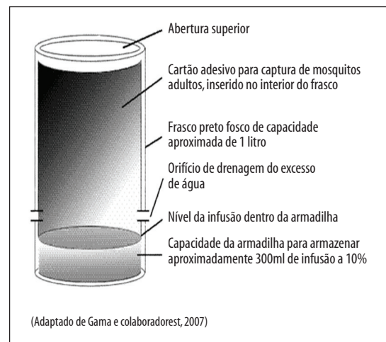
Figura 3 - Armadilha MosquiTRAP versão 1.0 utilizada nos experimentos de Pedro Leopoldo-MG. Brasil,
